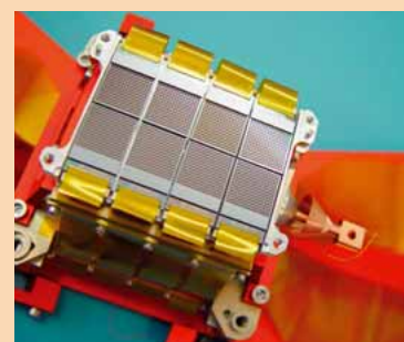
Le bolomètre est une sorte de thermomètre ultrasensible, capable de détecter d'infimes variations de température (quelques millièmes de degré). Ici, le plan focal bolométrique 32x64 pixels de l'instrument PACS.
